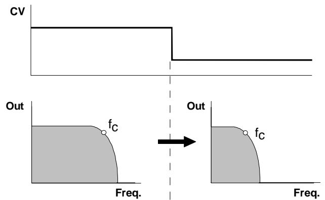
Abb. 1: Tiefpaß-Filtern weissen Rauschens
